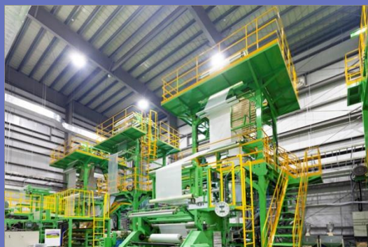
低密度ポリエチレン インフレ機
