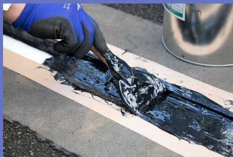
SMジョイント工法（橋梁補修）
