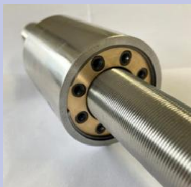
差動式ローラーネジ（外観）
