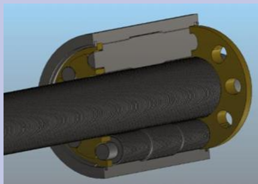
差動式ローラーネジの断面図
