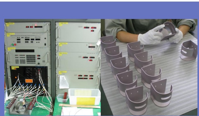
製品写真(電源トランス・精密板金)
