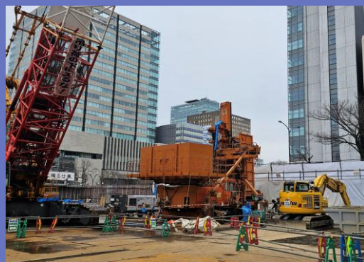
TRD工法 施工状況（当社保有機）
